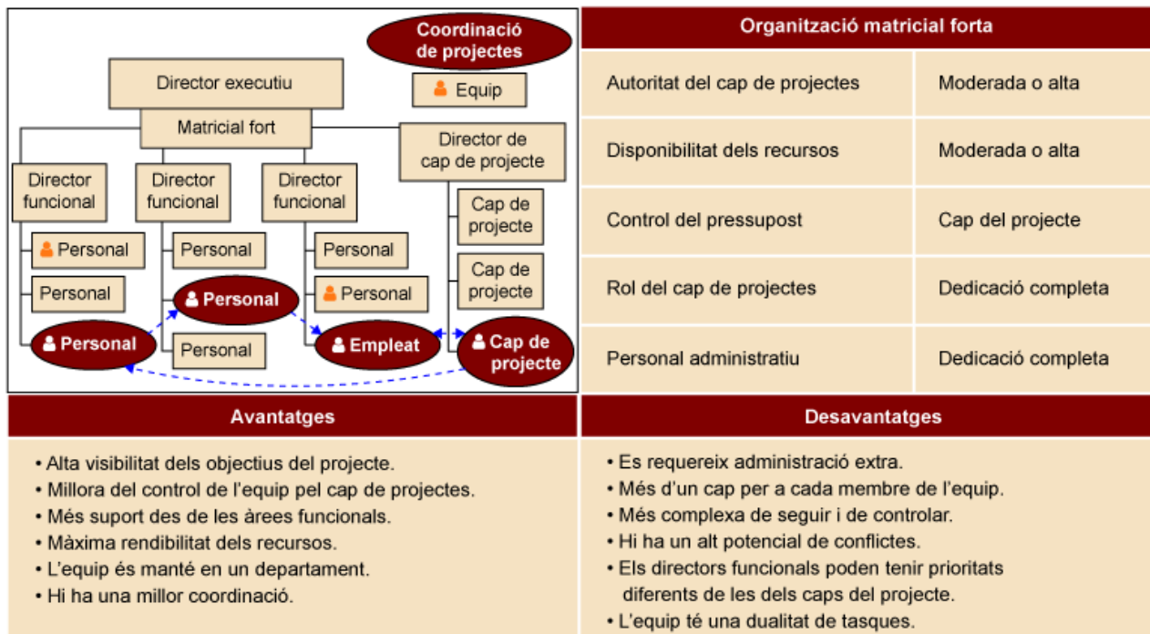
Figura 14. Organització matricial
