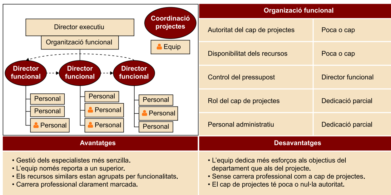
Figura 12. Organització funcional
