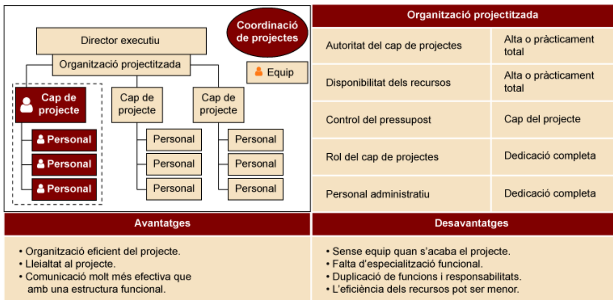
Figura 13. Organització projectitzada
